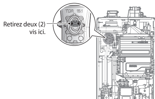
Figure 4. Accès à l'orifice d'évacuation des gaz dans le ventilateur
