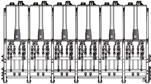
[Configuration modulaire avec système de supports Navien]
